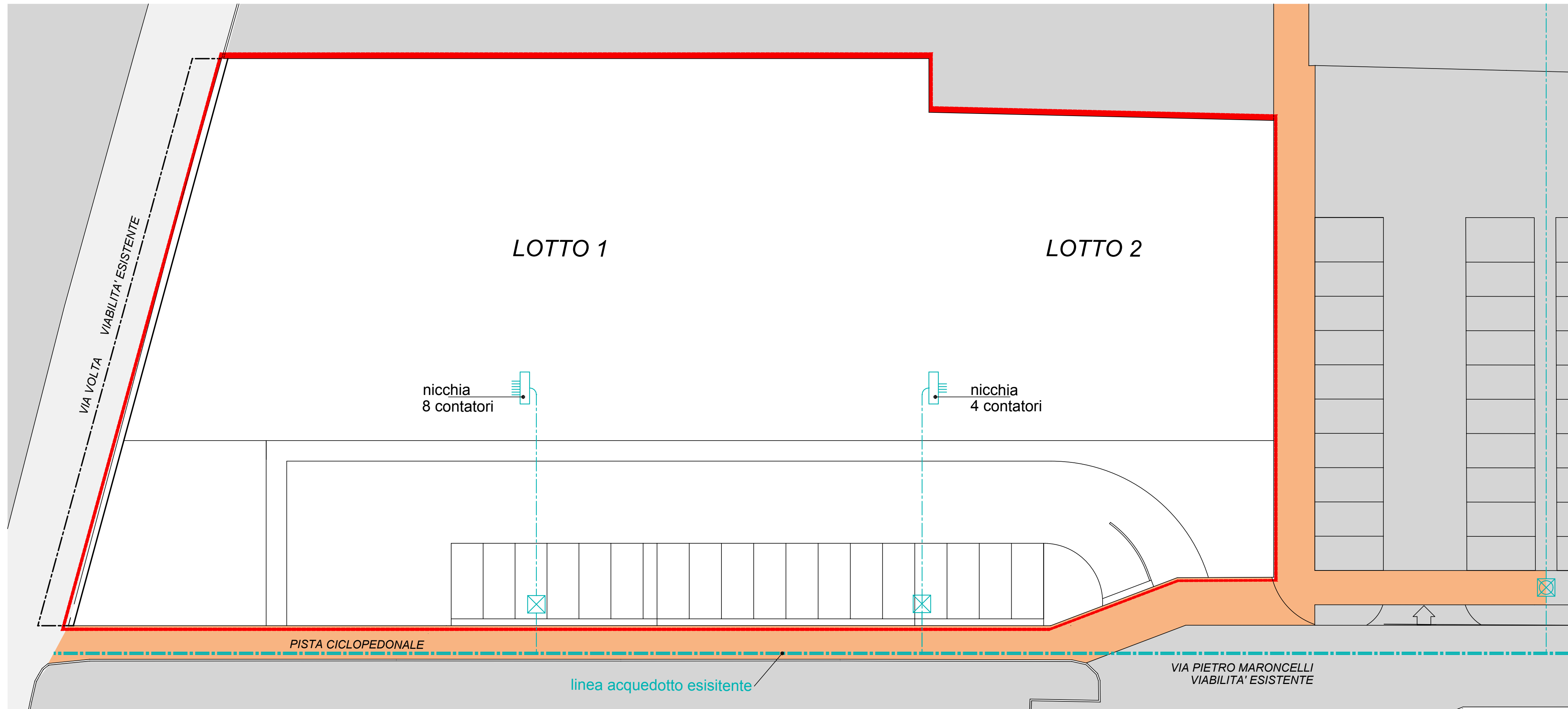
PLANIMETRIA RETE DISTRIBUZIONE ACQUEDOTTO 1:200
